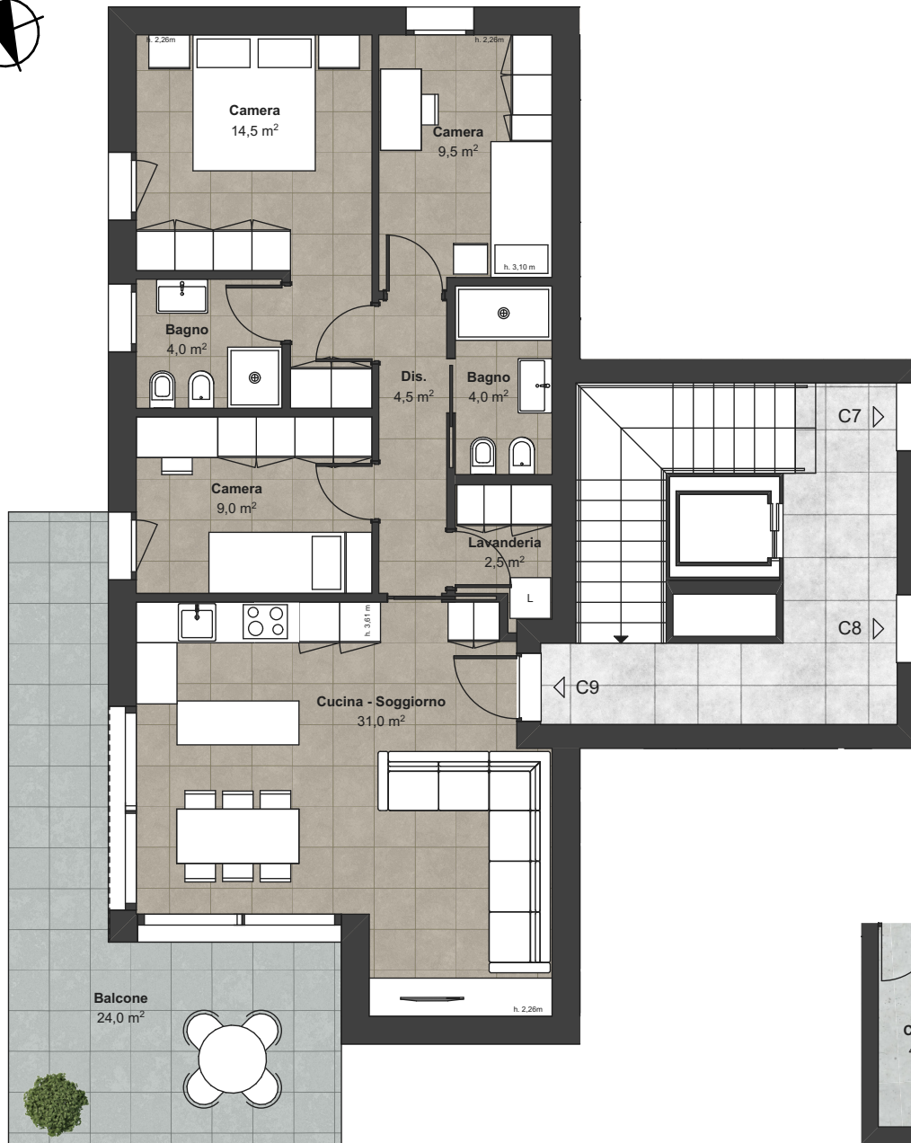
Piano Secondo (Scala 1:100)
